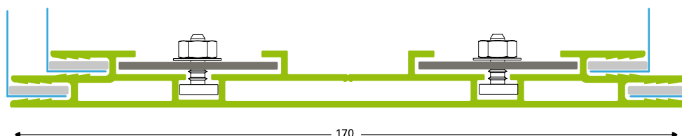
Intex Lux 170 Lightbox, 2-seitig eloxiert
